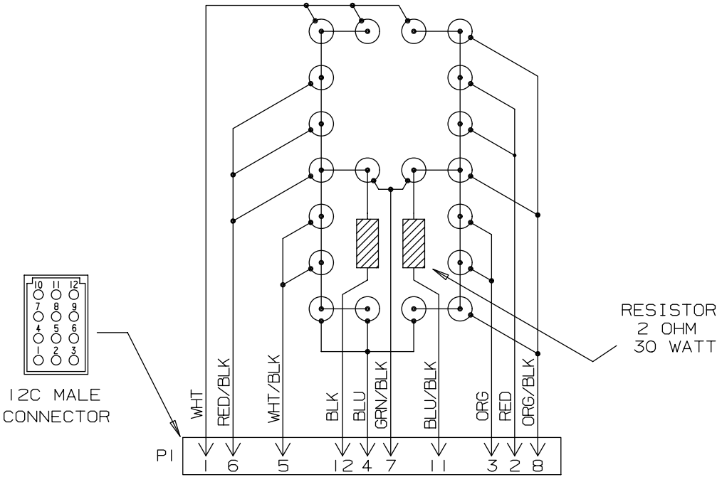
0-9 FIGUREGRAM WIRING
